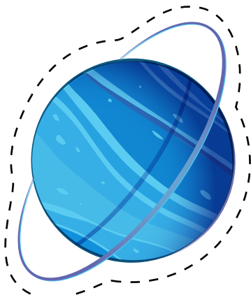
7. Uranus
