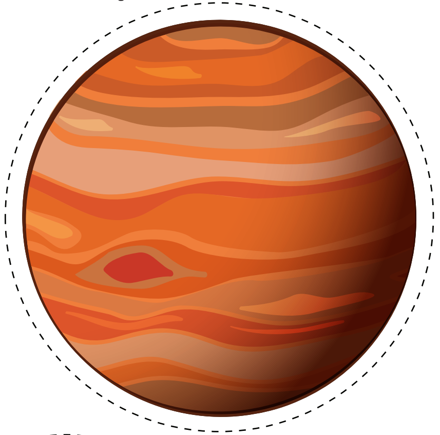
5. Jupiter
